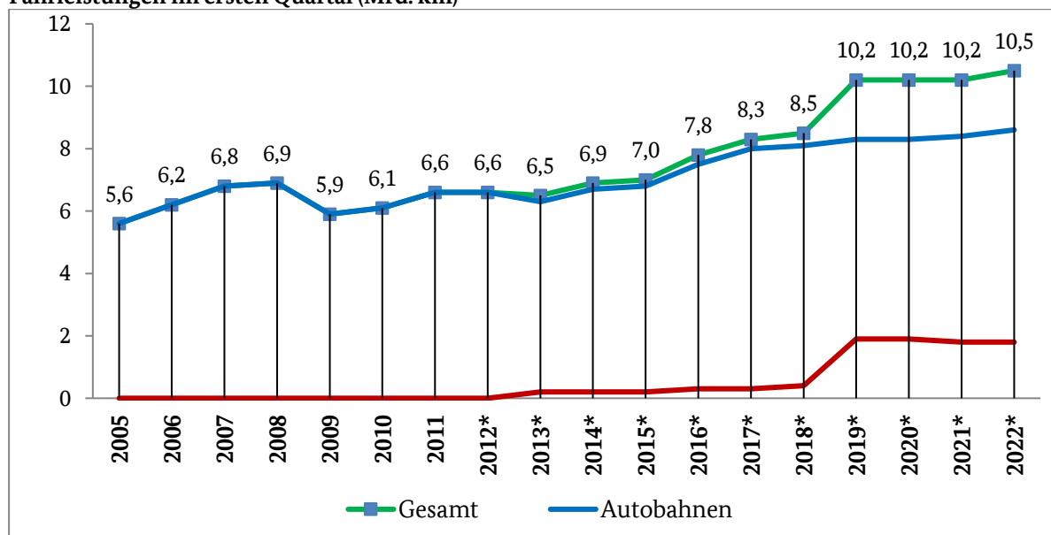
Fahrleistungen im ersten Quartal (Mrd. km)
